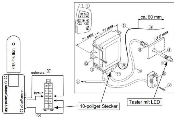
Abbildung 2: Anschluss des MicroGuard-USB Moduls an die Leitungen am Heizgerät (siehe Beschreibung).
