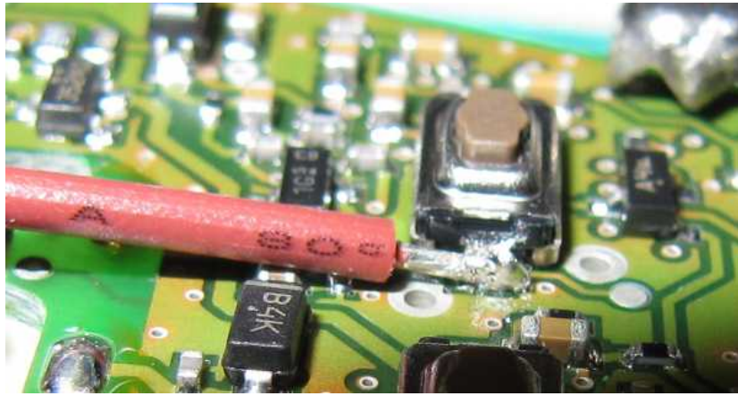
Abbildung 2: Sauberer Lötspunkt an der Seite des „ON“ Tasters
