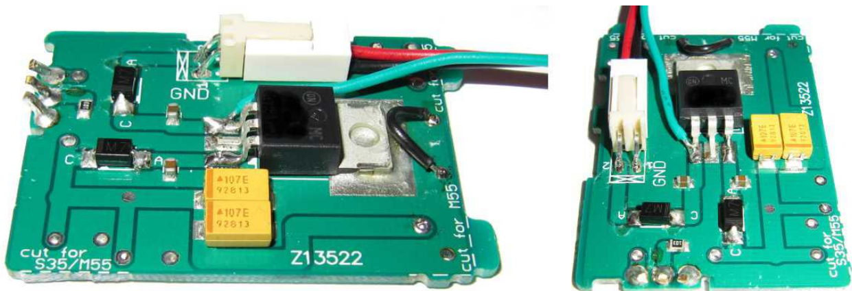
Abbildung 5: Anschluss der grünen Leitung für +12V am Akku-Ersatz
