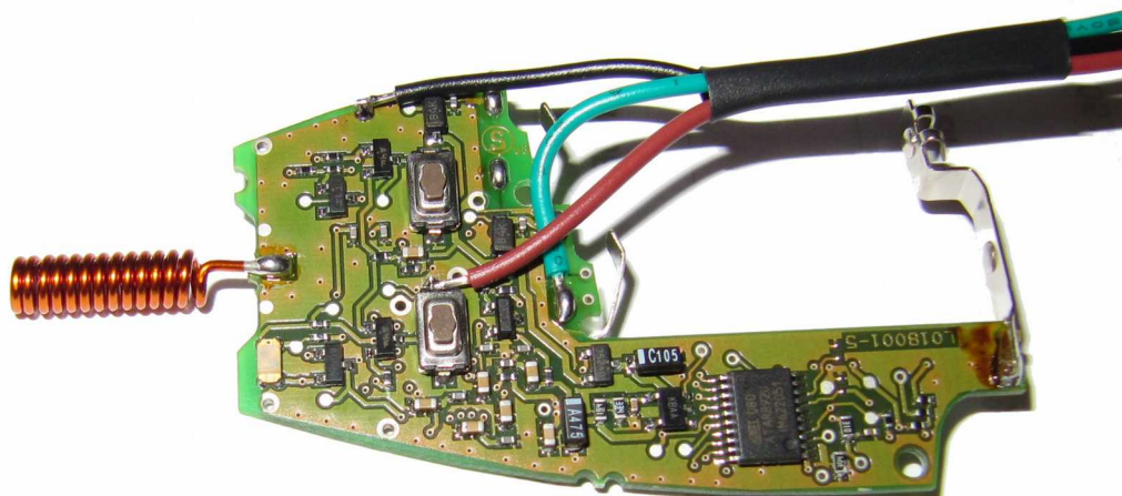
Abbildung 3: Steuerleitung (braun) und Versorgungsleitungen (grün: +12V; schwarz: Masse)
