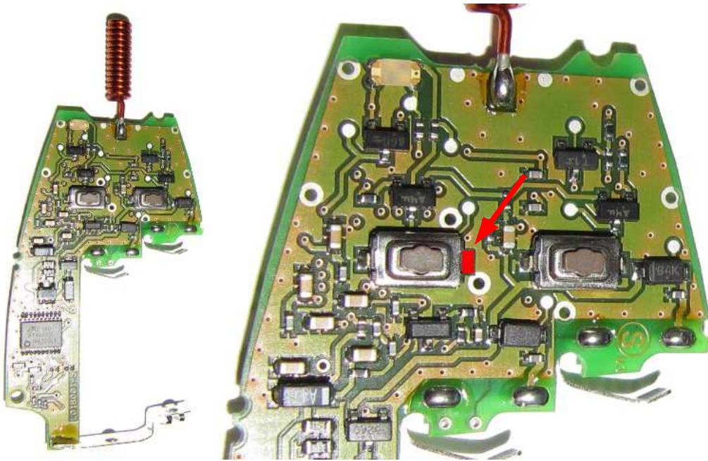
Abbildung 1: Anschlusspunkt (roter Pfeil) für die MG Steuerleitung (braun, nicht im Bild dargestellt)
