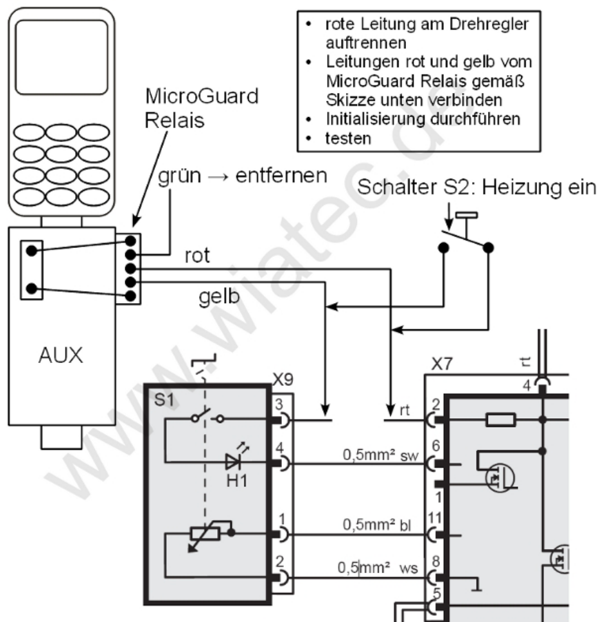
Abbildung 1: Schematische Darstellung des Anschlusses von Steuermodul und Standheizungssteuerung
